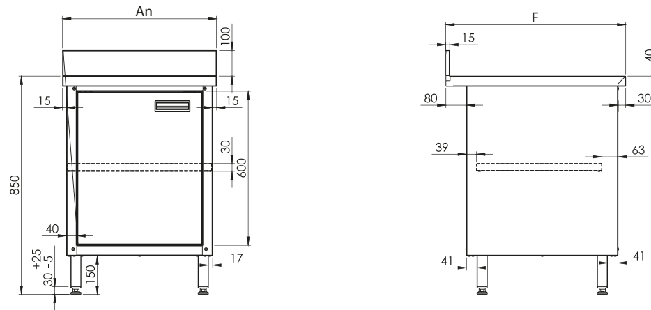
014 MESA MURAL CON PUERTAS BATIENTES
