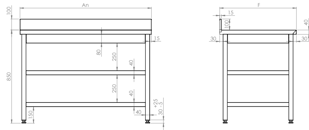
006 MESA DE PARED CON 2 ESTANTES
