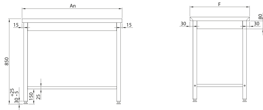
008 MESA CENTRAL SIN ESTANTE
