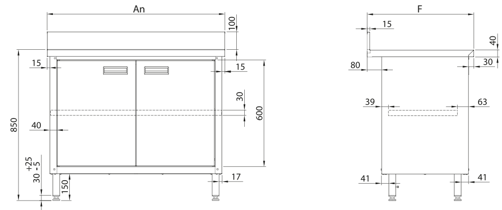
015 MESA MURAL CON ARMARIO Y PUERTAS ABATIBLES
