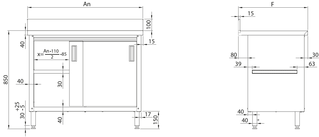
018 MESA MURAL CON ARMARIO Y PUERTAS CORREDIZAS
