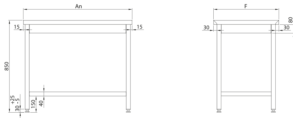
010 MESA CENTRAL CON ESTANTE
