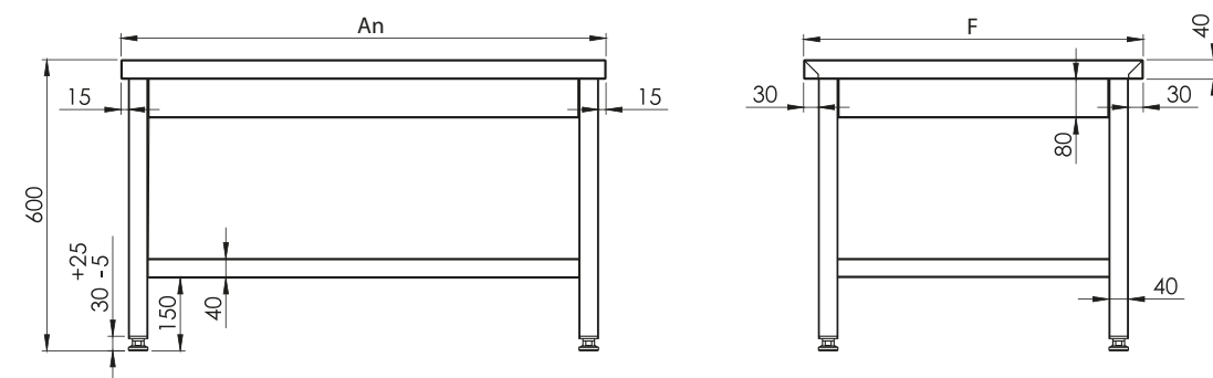
425 MESA BAJA CENTRAL CON ESTANTE
